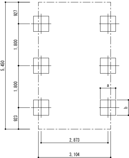
■基礎配置図
